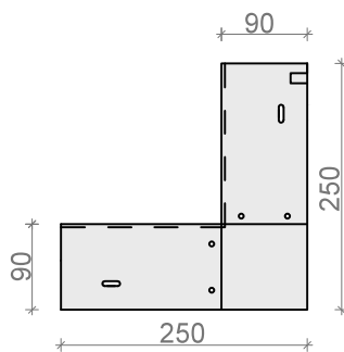
NAROŻNIK WEWN. 90° NK 95ALw, NK 95Sw
