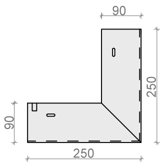
NAROŻNIK ZEWN. 90° NK 95ALz, NK 95Sz
