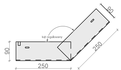
NAROŻNIK ZEWN. regulowany NK 95ALzR, NK 95SzR
